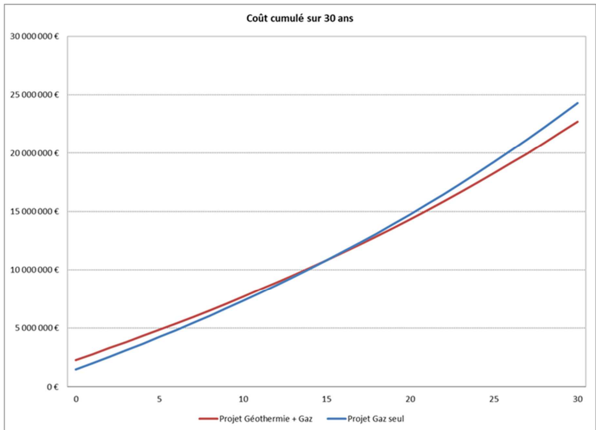
Figure 2 : Coût comparatif sur 30 ans de la solution « géothermie + gaz » et de la solution « gaz seul »
