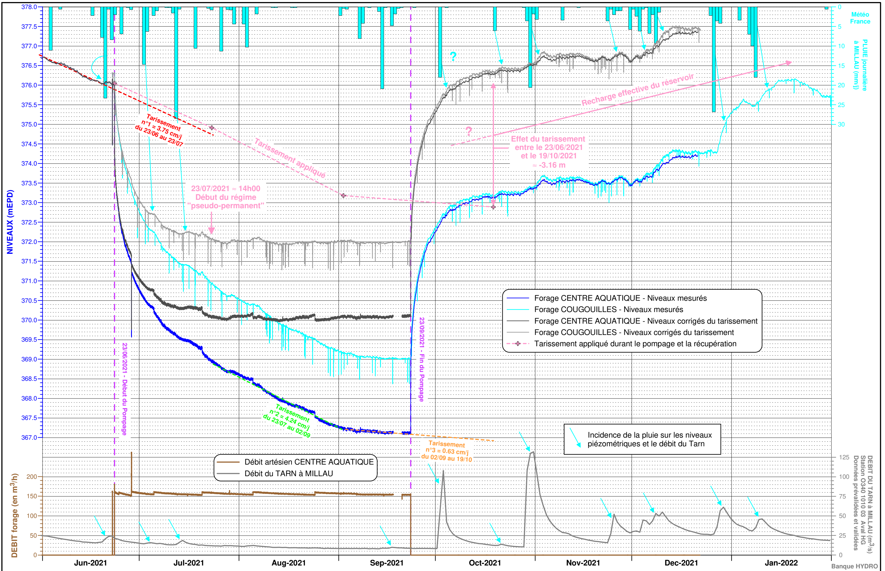
SUIVI HYDRAULIQUE DU 01/06 AU 22/12/2021 FORAGES DU CENTRE AQUATIQUE ET DE COUGOUILLES PLUVIOMETRIE ET DEBIT DU TARN A MILLAU
