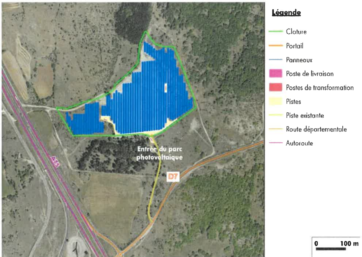
Carte extraite de l'étude d'impact qui présente l'ensemble des équipements du projet page 21 réalisée par ARTIFEX – source BDORTHO IGN
