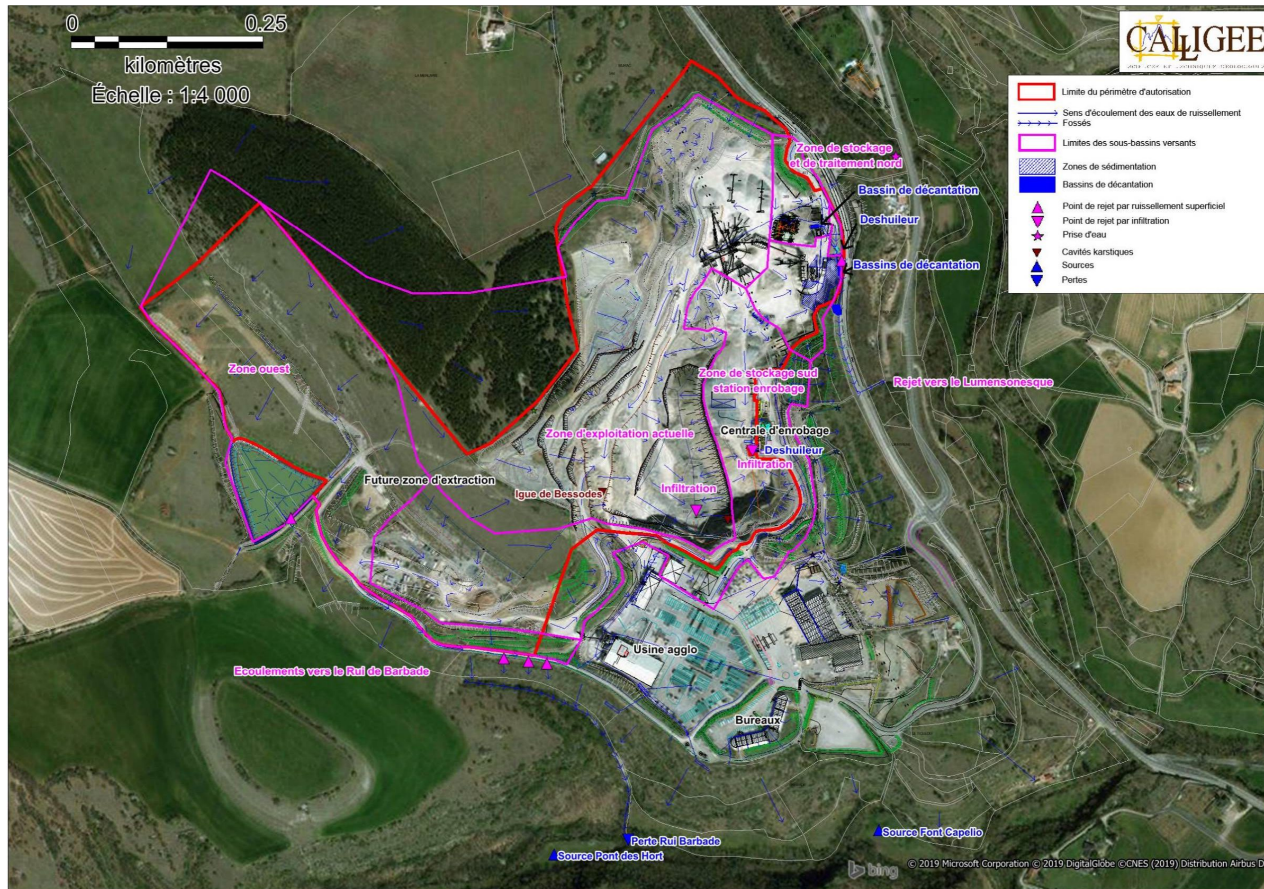
Figure 14 : Découpage des sous-bassins versants pour la configuration actuelle de l'exploitation (source : rapport CALLIGEE – octobre 2019 – Figure 11 échelle non conservée)
